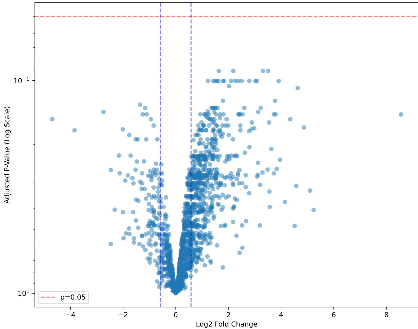
Volcano Plot: D11 - T0
